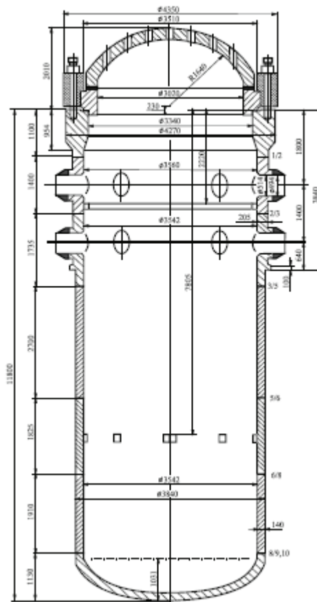
1. ábra. A reaktortartály hosszmet szete a főbb méretekkel.
