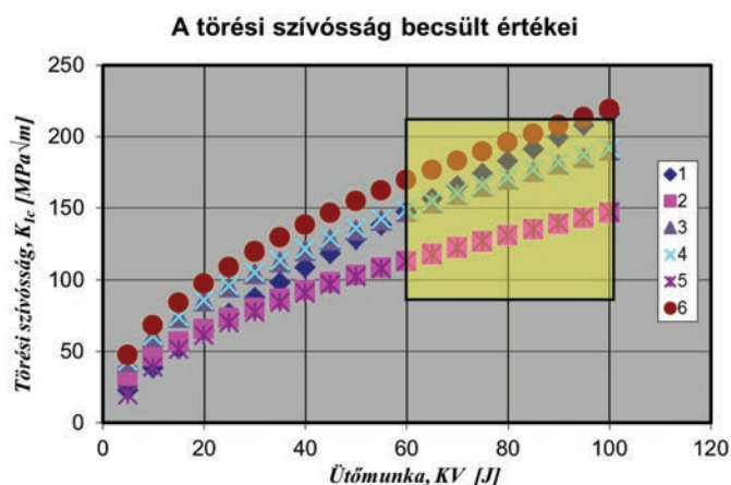
5. ábra. A K_{Ic} becsült értékei a Charpy-V próbatesteken mért ütésmunka függvényében
